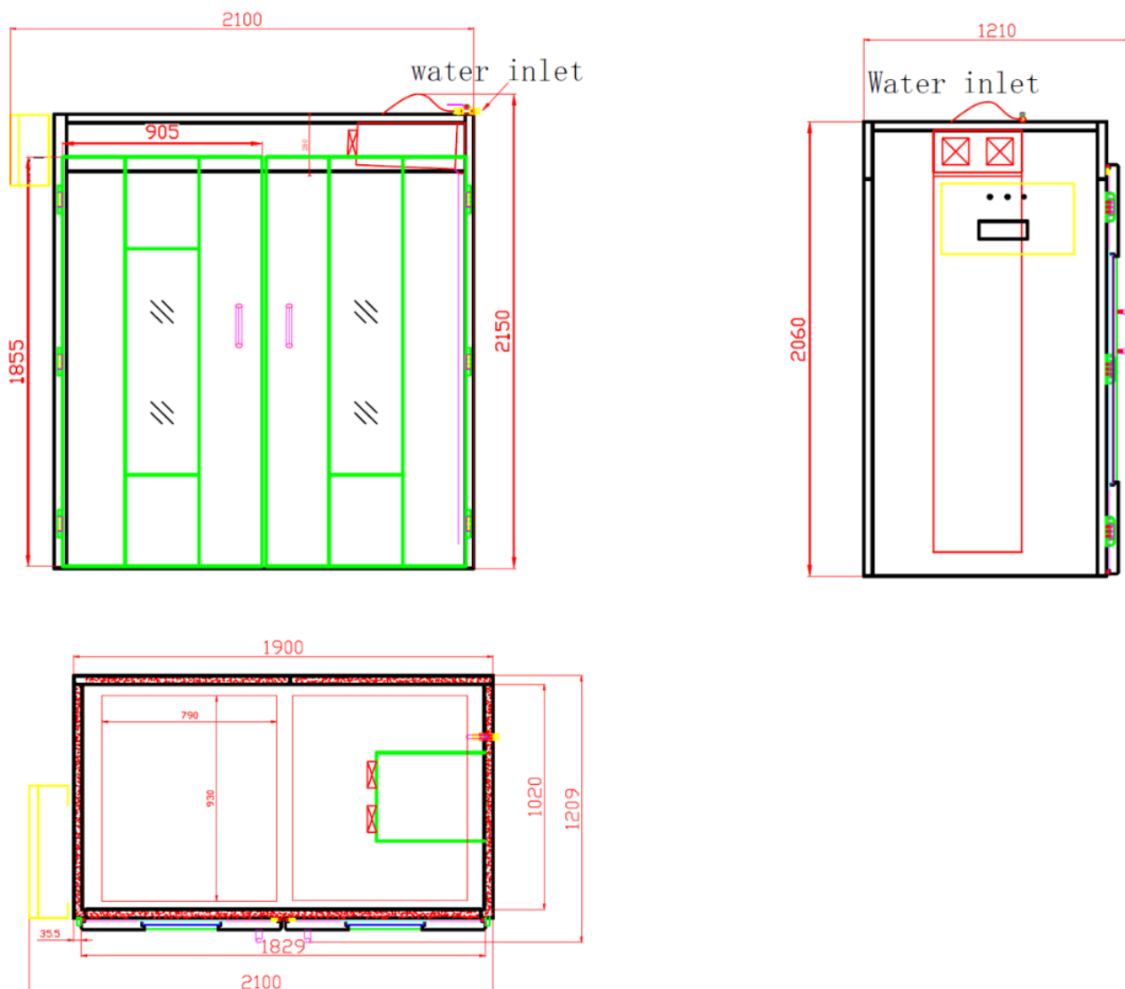
Габаритный чертеж MIRATEK PRF-2 (2 тележки 600x800)
